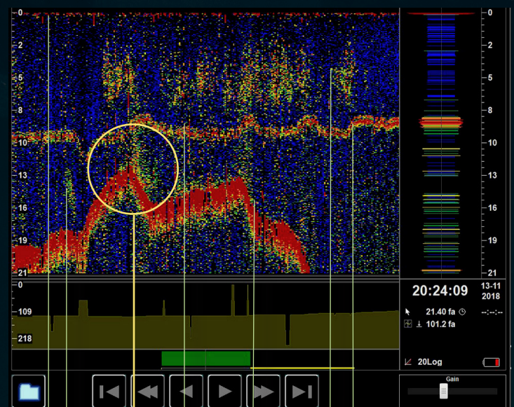
Визуализация объектов лова относительно трала
