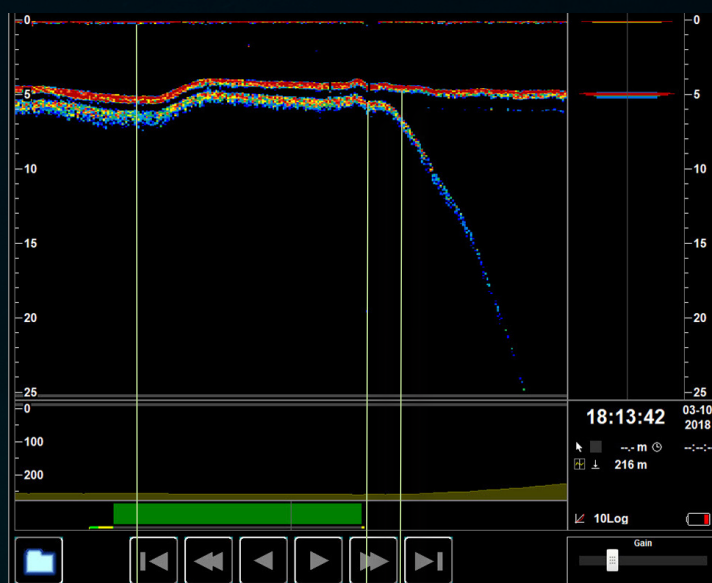
Визуализация раскрытия трала
